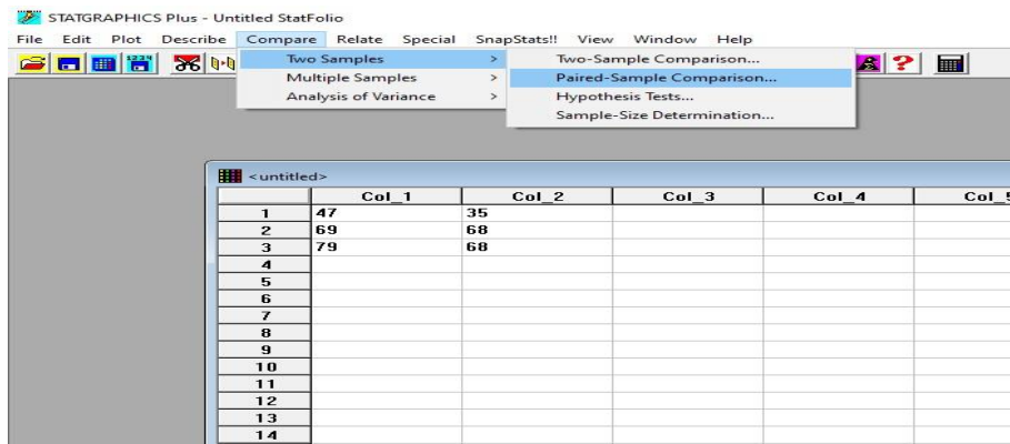
Figura 2.7: Paso 1 del procedimiento para determinar diferencias significativas entre los datos para análisis de muestras pareadas.
