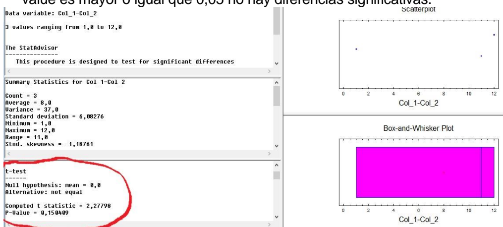
Figura 2.10: Paso 4 del procedimiento para determinar diferencias significativas entre los datos para análisis de muestras pareadas.
