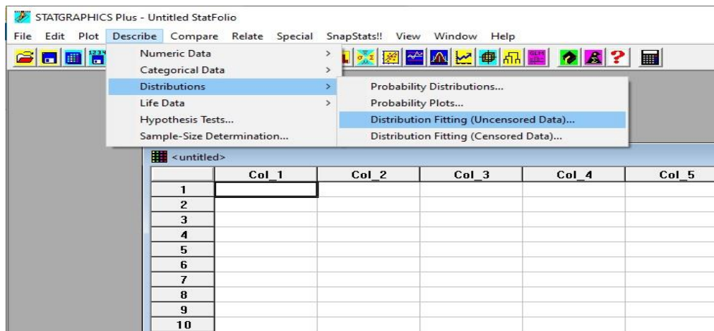
Figura 2.2: Paso 1 del procedimiento para determinar normalidad de los datos.
