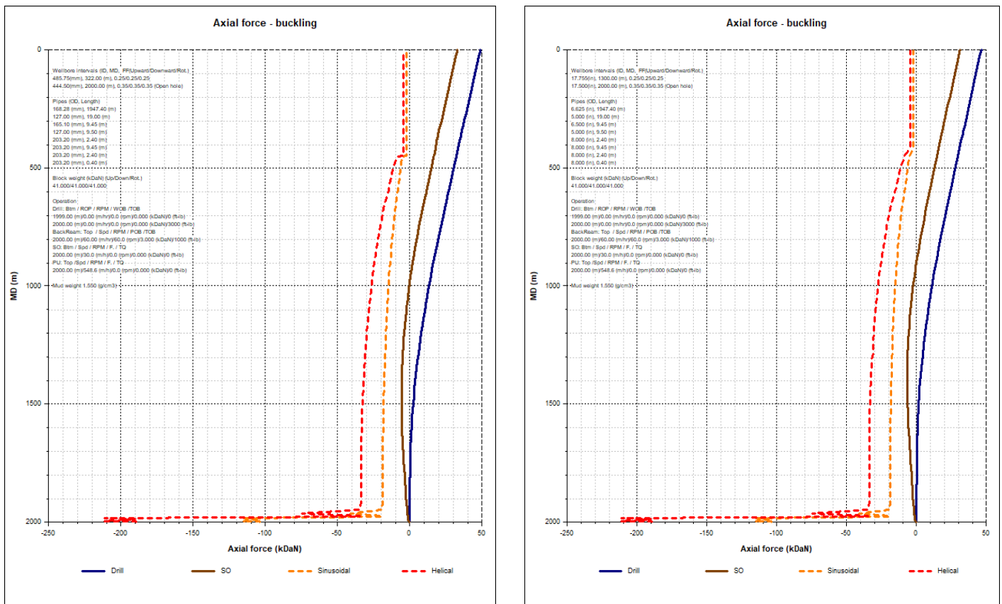
Figura 3.10 Axial Force- Buckling en la construcción en una y dos etapas.
