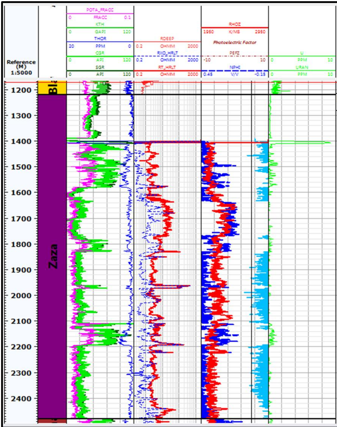
Fig. 3.1: Intervalo correspondiente al Complejo Ofiolítico (Formación Zaza), donde se observa la existencia de paquetes diferentes dentro de la misma formación.
