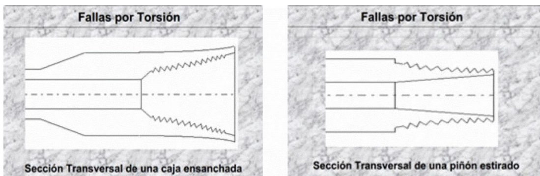
Figura 1.2 Fallas por torsión
