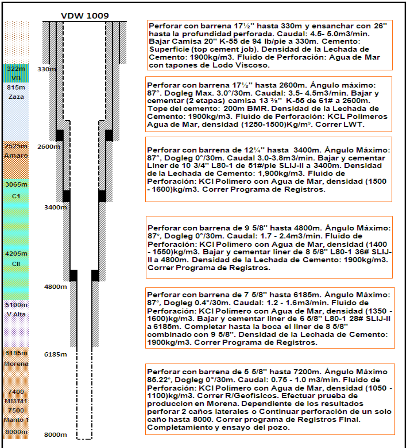
Figura 2.1 Construcción del Pozo. Resumen por Etapas
