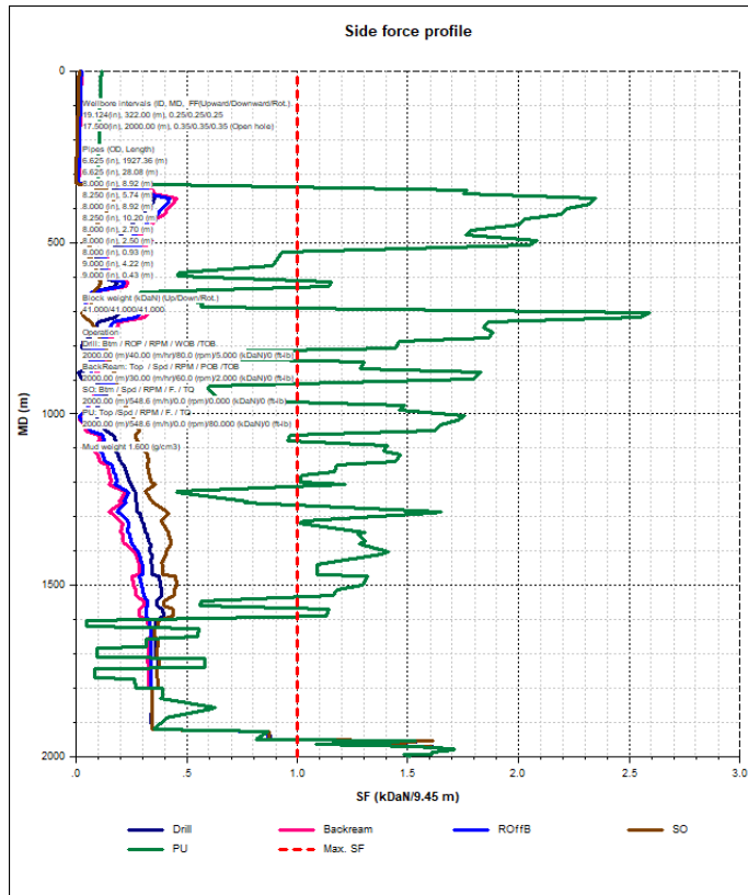
Fig. 3.8 Esfuerzos laterales
