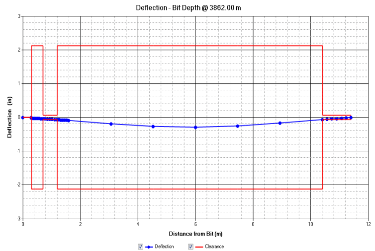
Figura3.14 Deformaciones de la BHA (BHA original y BHA modificada)
