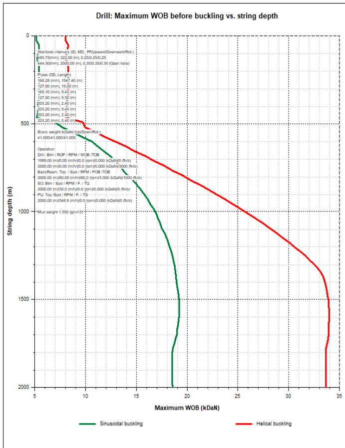
Figura 3.11 Máximo WOB antes del Buckling en la construcción en una y dos etapas
