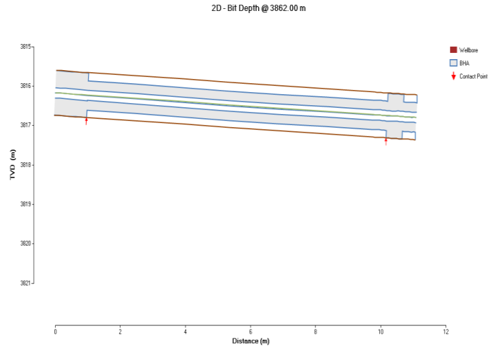
Figura 3.13 Puntos de contacto entre la BHA y el caño (BHA original y BHA modificada)
