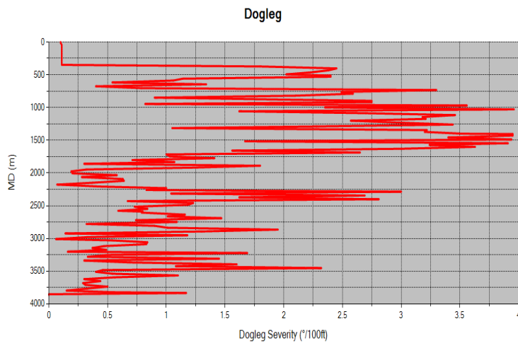
Figura3.12 Geometría del pozo
