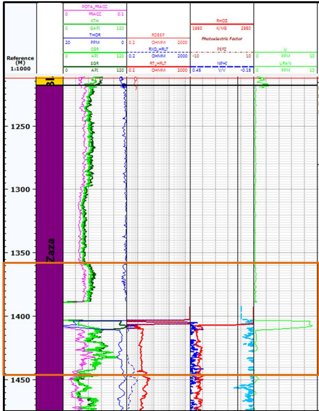
Fig. 3.2 Imagen de los registros geofísicos en el intervalo correspondiente a los dos primeros paquetes descritos. (Se muestra con rectángulo naranja el segundo paquete descrito, correspondiente a ofiolitas serpentinizadas)
